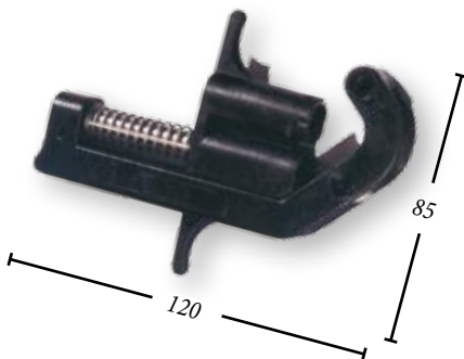
Bộ dụng cụ lột bán dẫn ngoài - AV6410
