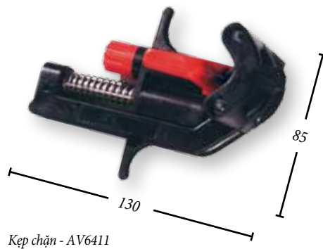
Kẹp chặn - AV6411
